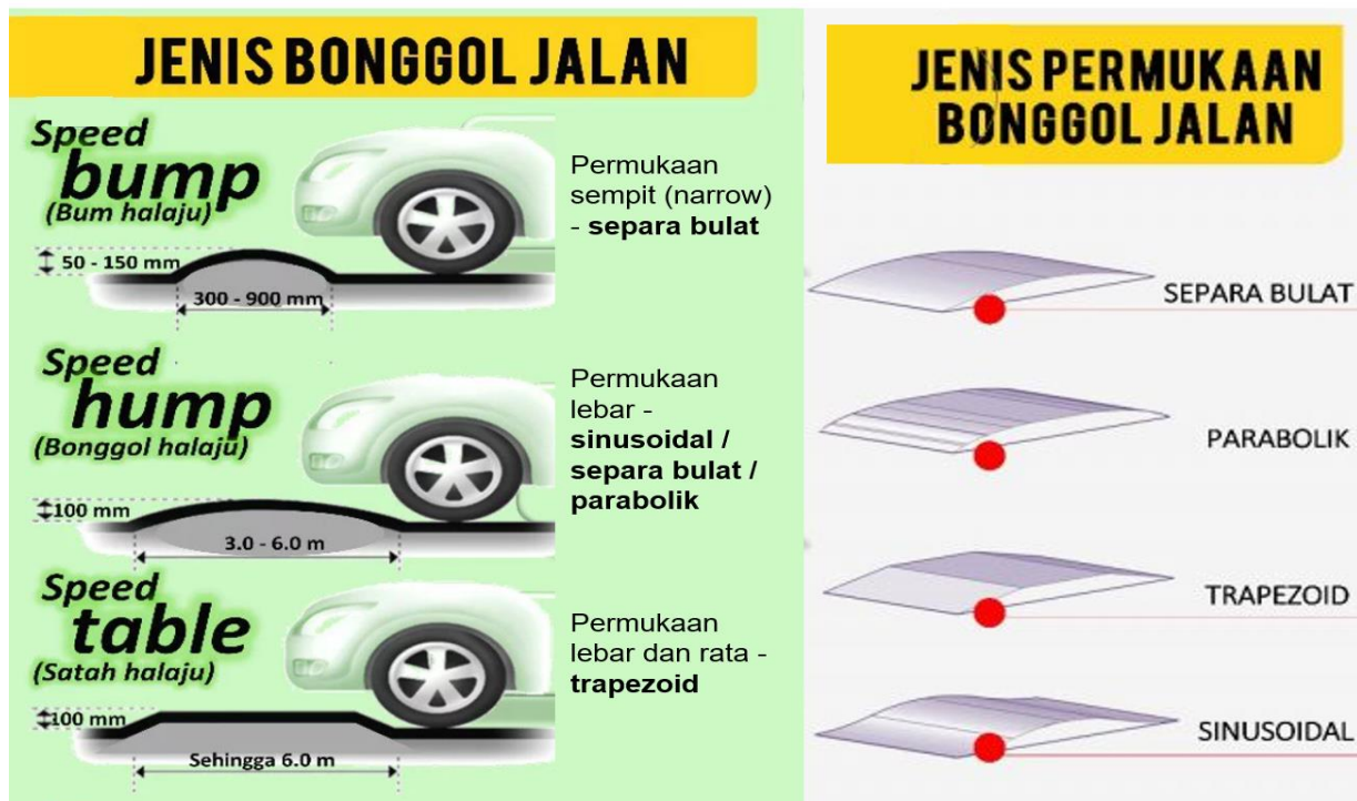
Rajah 16: Perincian jenis bonggol jalan
